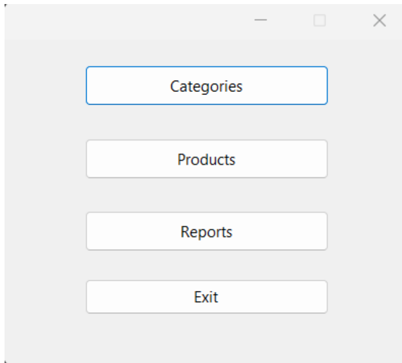
Рисунок 2 – Меню программы
